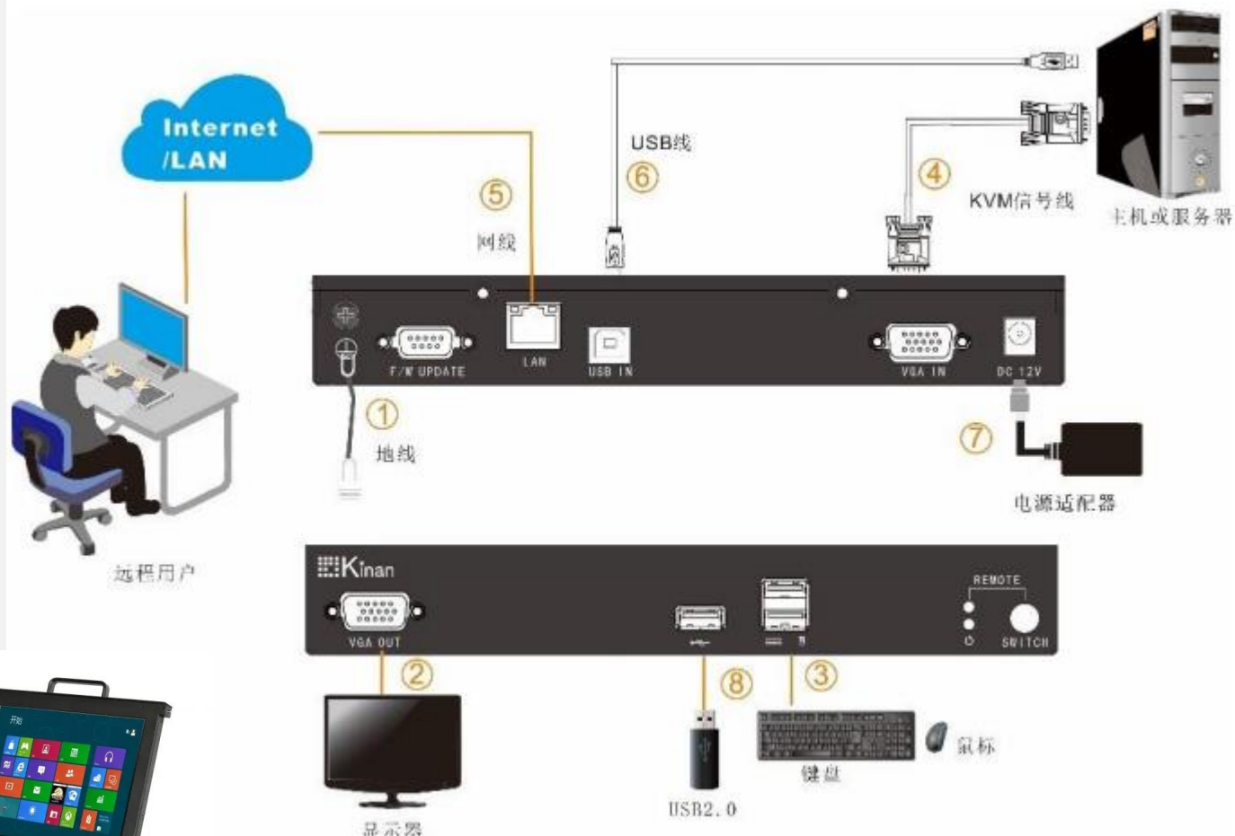
设备接线示意图
